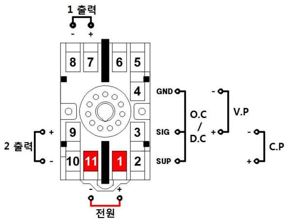
[2 출력 (11핀)]
