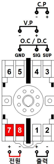
[1 출력 (8핀)]
