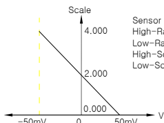
EX2) Input Range : -50~+50mV Display Scale : 4.000~0.000
